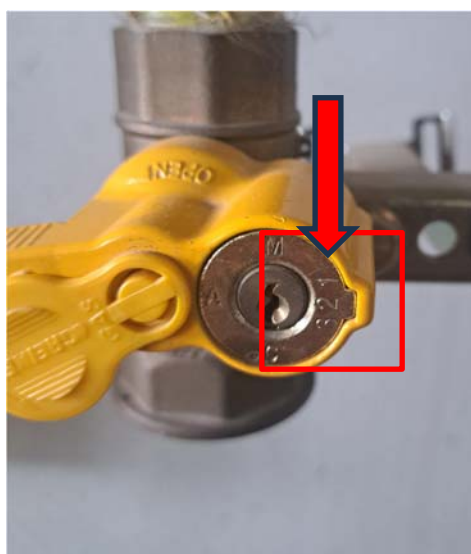
numero chiave stampigliato sul nottolino
